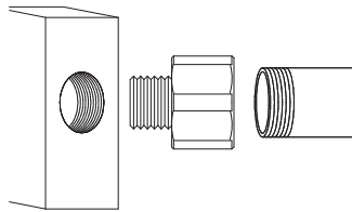
防爆構造接続箱 逆アダプター 防爆構造附属品
